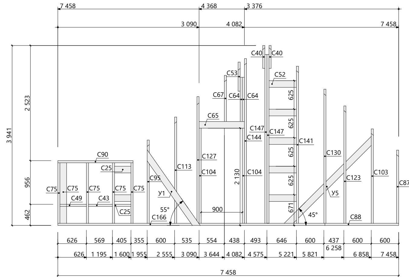
Схема сборки СтК 2.07
