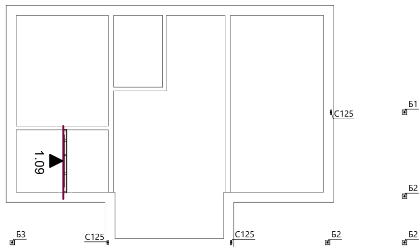
План-схема СтК 1.09
