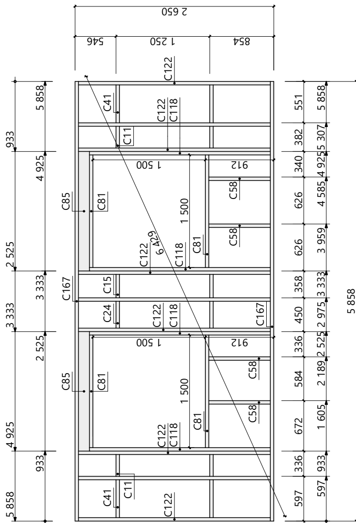
Схема сборки СтК 1.03
