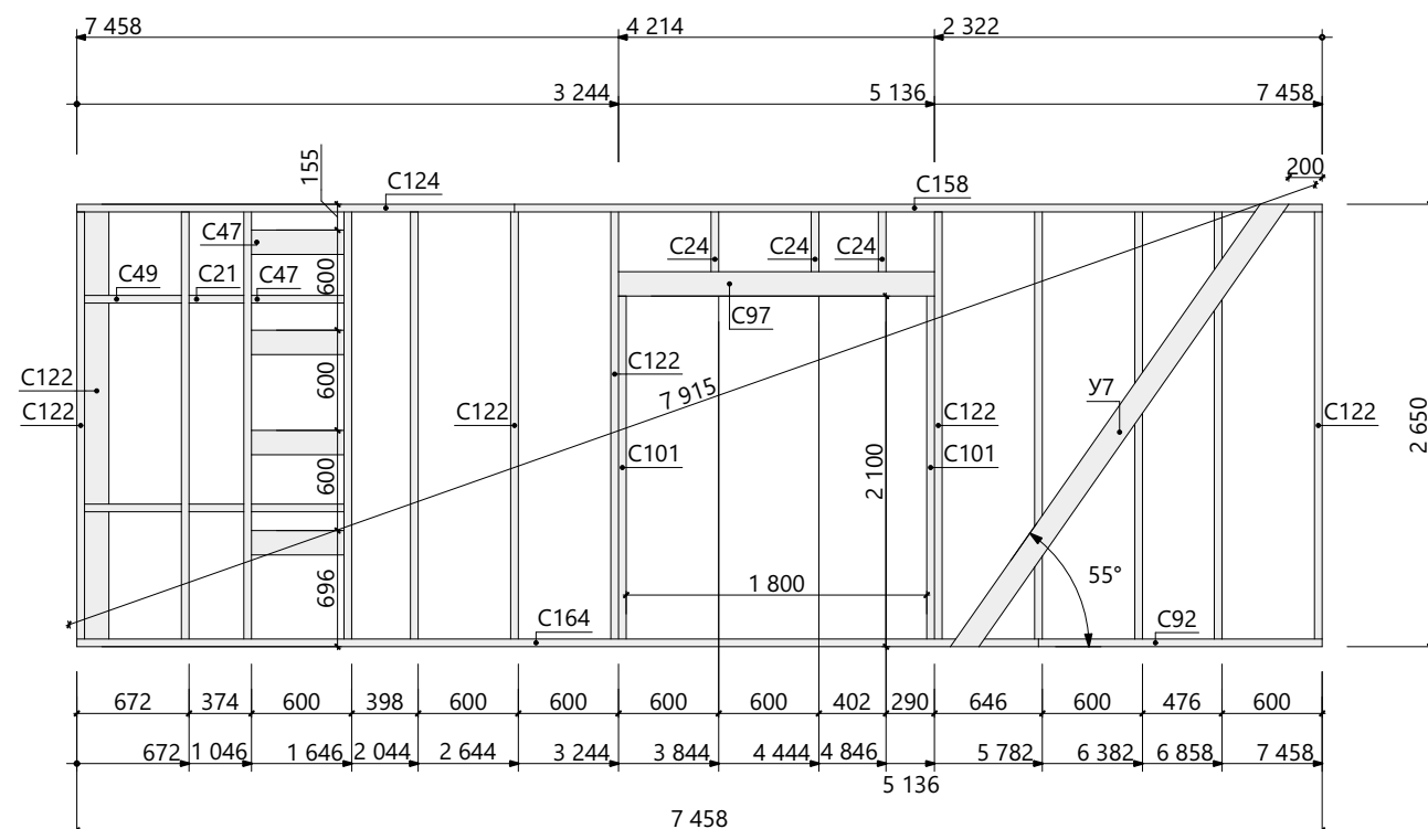
Схема сборки СтК 1.05
