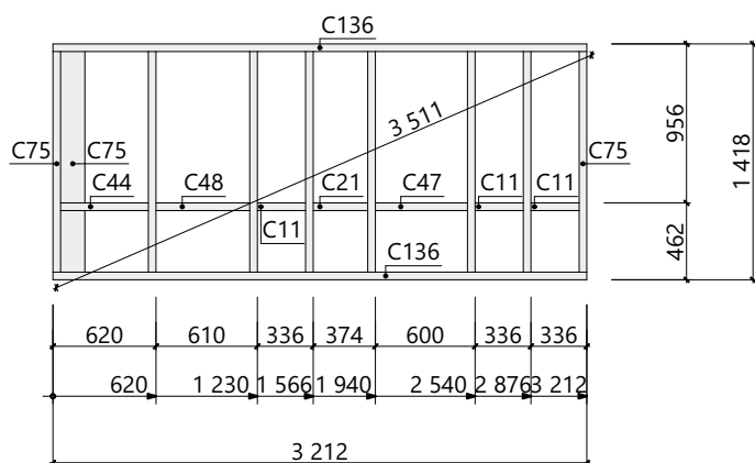
Схема сборки СтК 2.08
