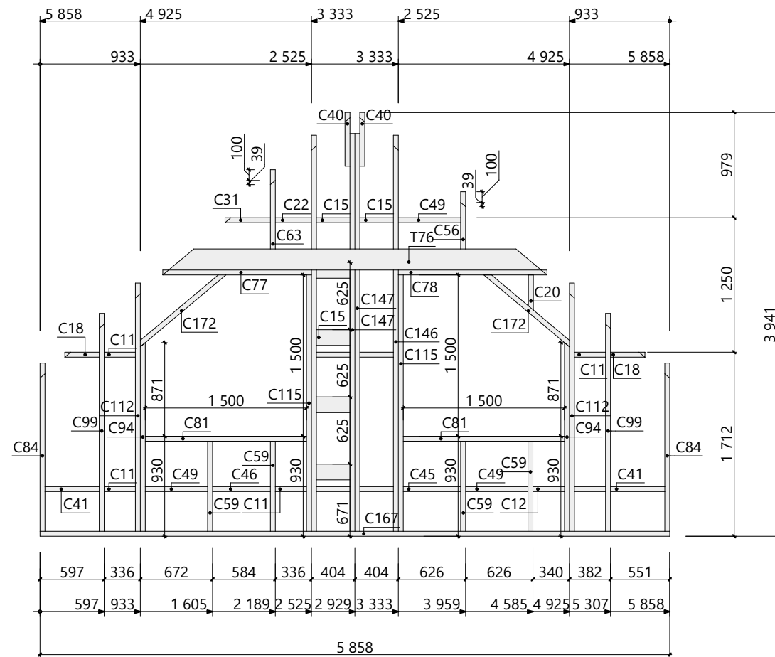
Схема сборки СтК 2.03
