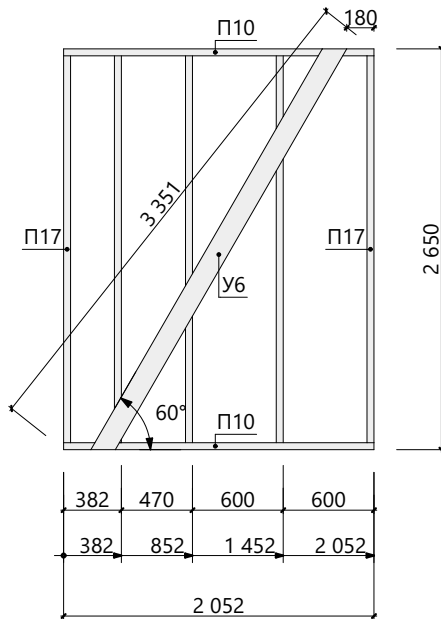
Схема сборки СтК 1.09
