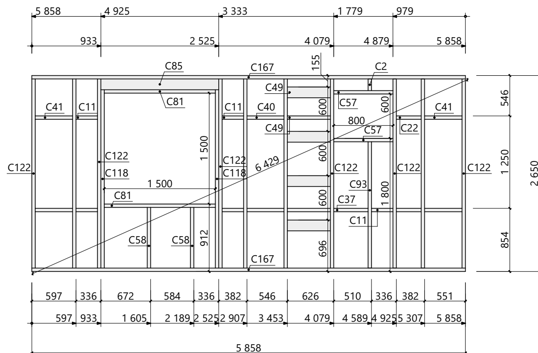
Схема сборки СтК 1.01
