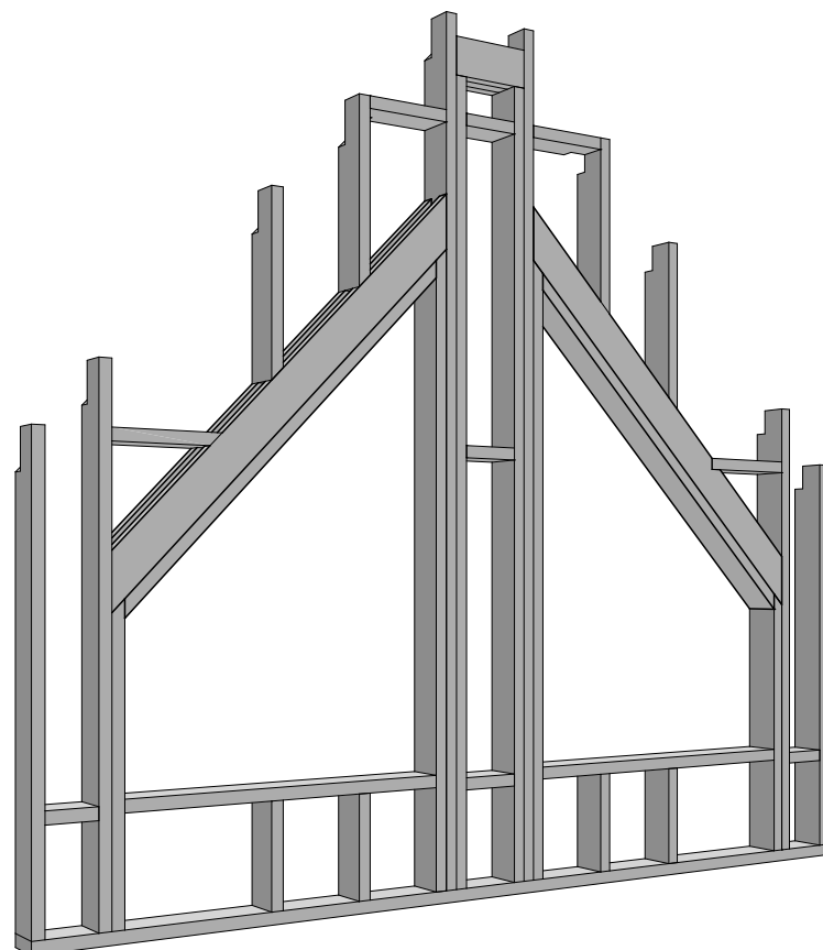
3-д Вид СтК 2.06
