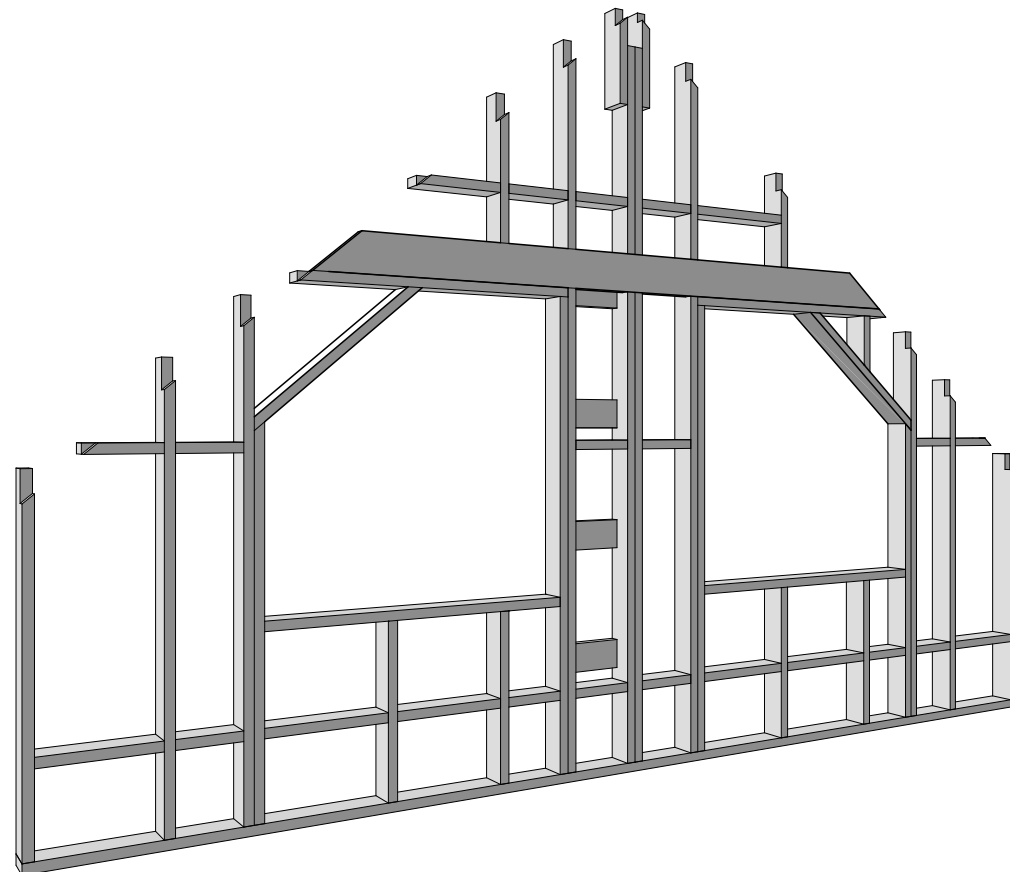
3-д Вид СтК 2.03
