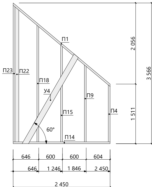
Схема сборки СтК 2.10
