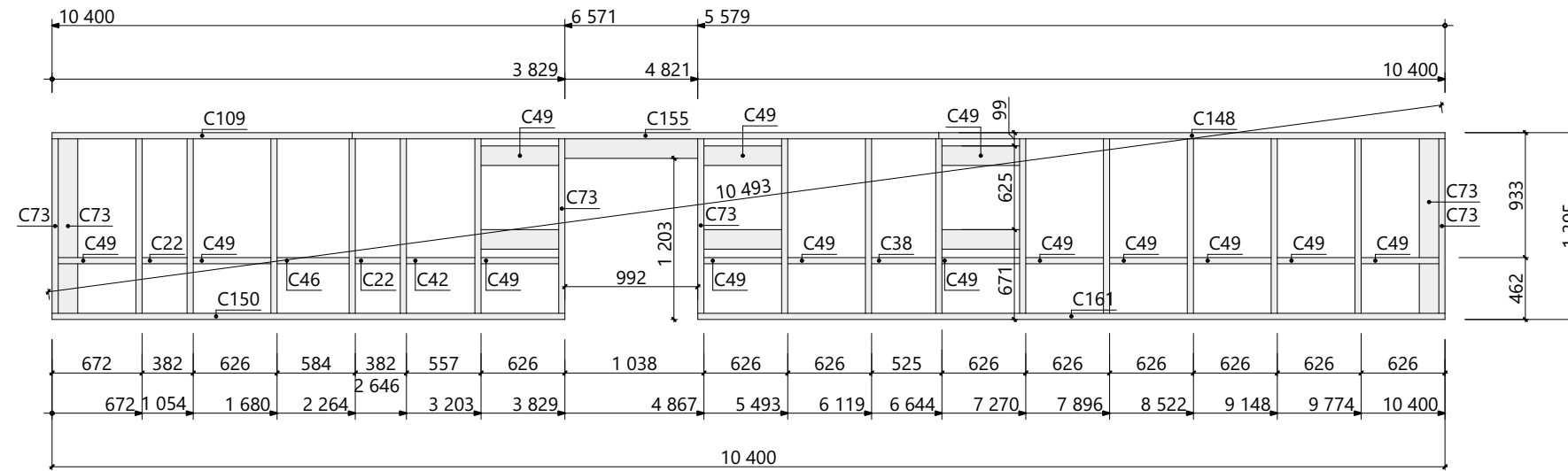
Схема сборки СтК 2.02
