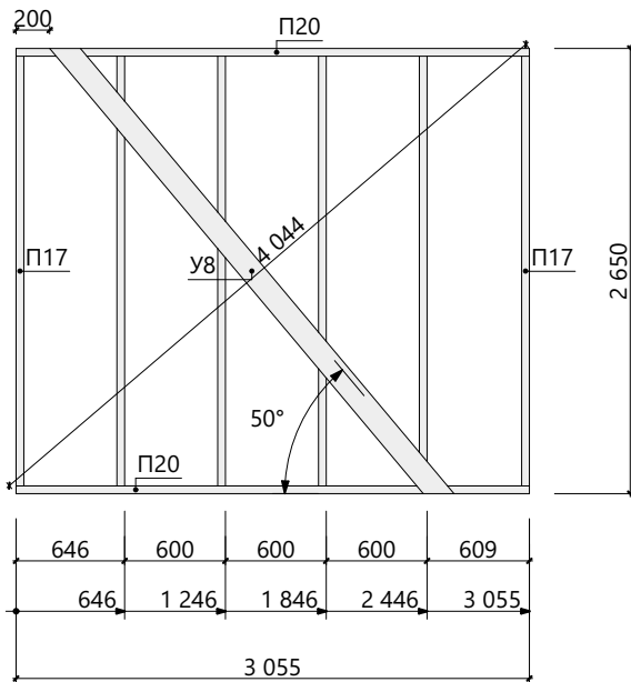
Схема сборки СтК 2.11
