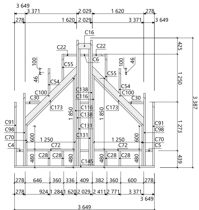
Схема сборки СтК 2.06
