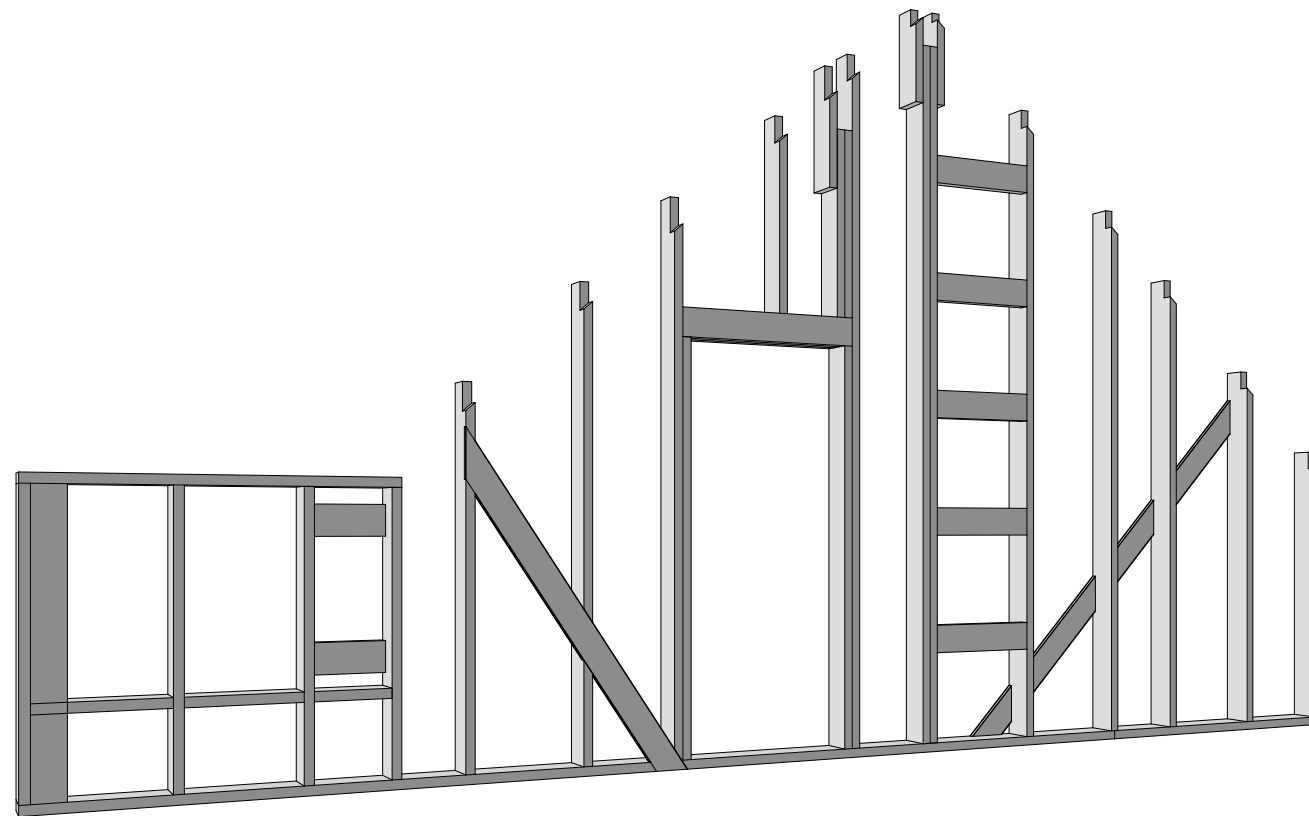
3-д Вид СтК 2.07
